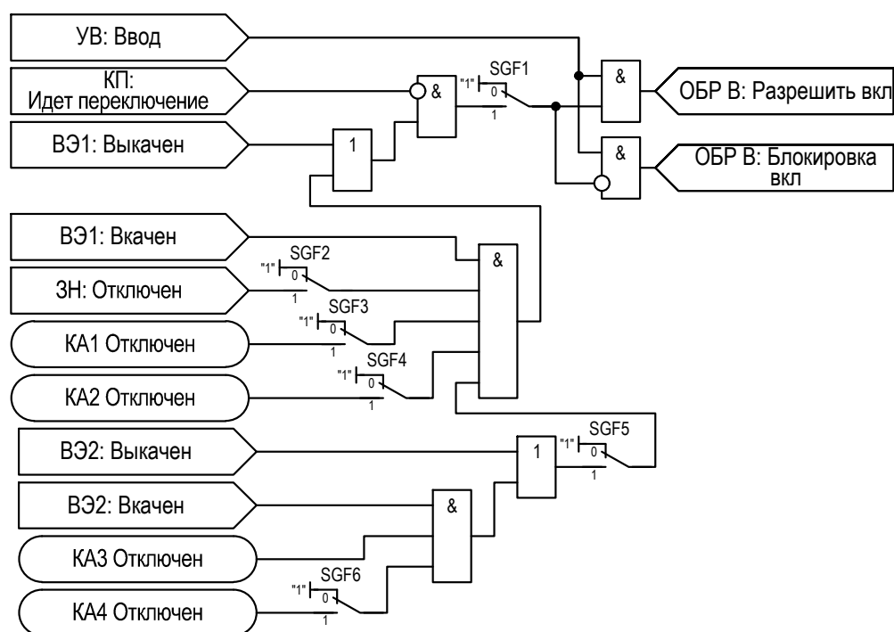
Рисунок 2.52 – Функциональная схема «ОБР В»
