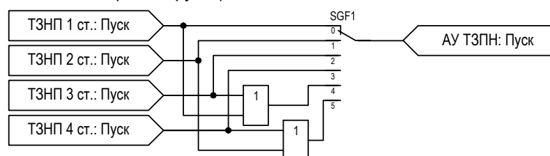
Рисунок 2.32 – Функциональная схема АУ ТЗНП
