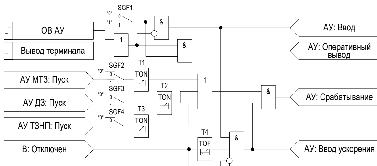
Рисунок 2.13 – Функциональная схема «АУ»
