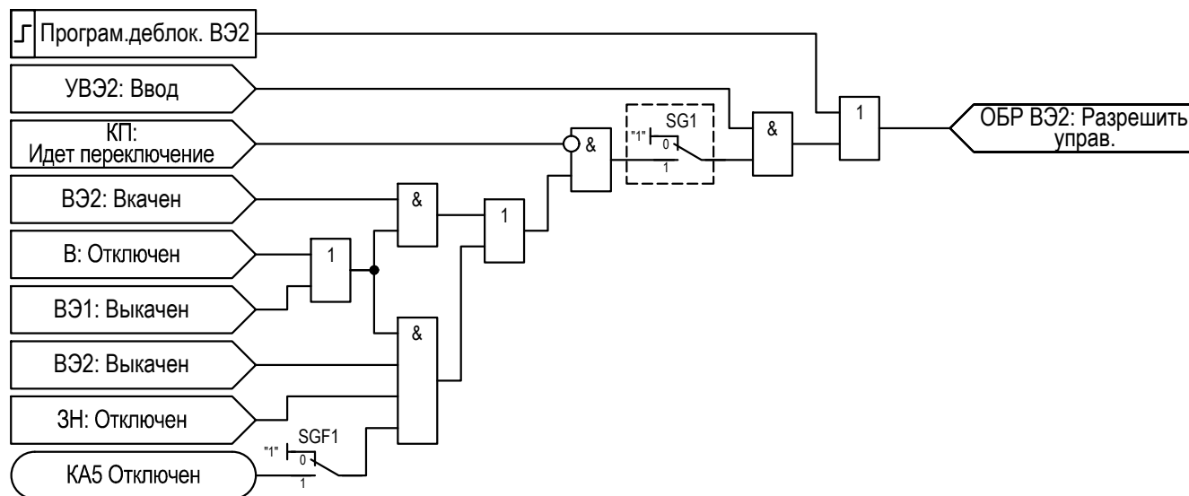
Рисунок 2.55 – Функциональная схема «ОБР ВЭ2»
