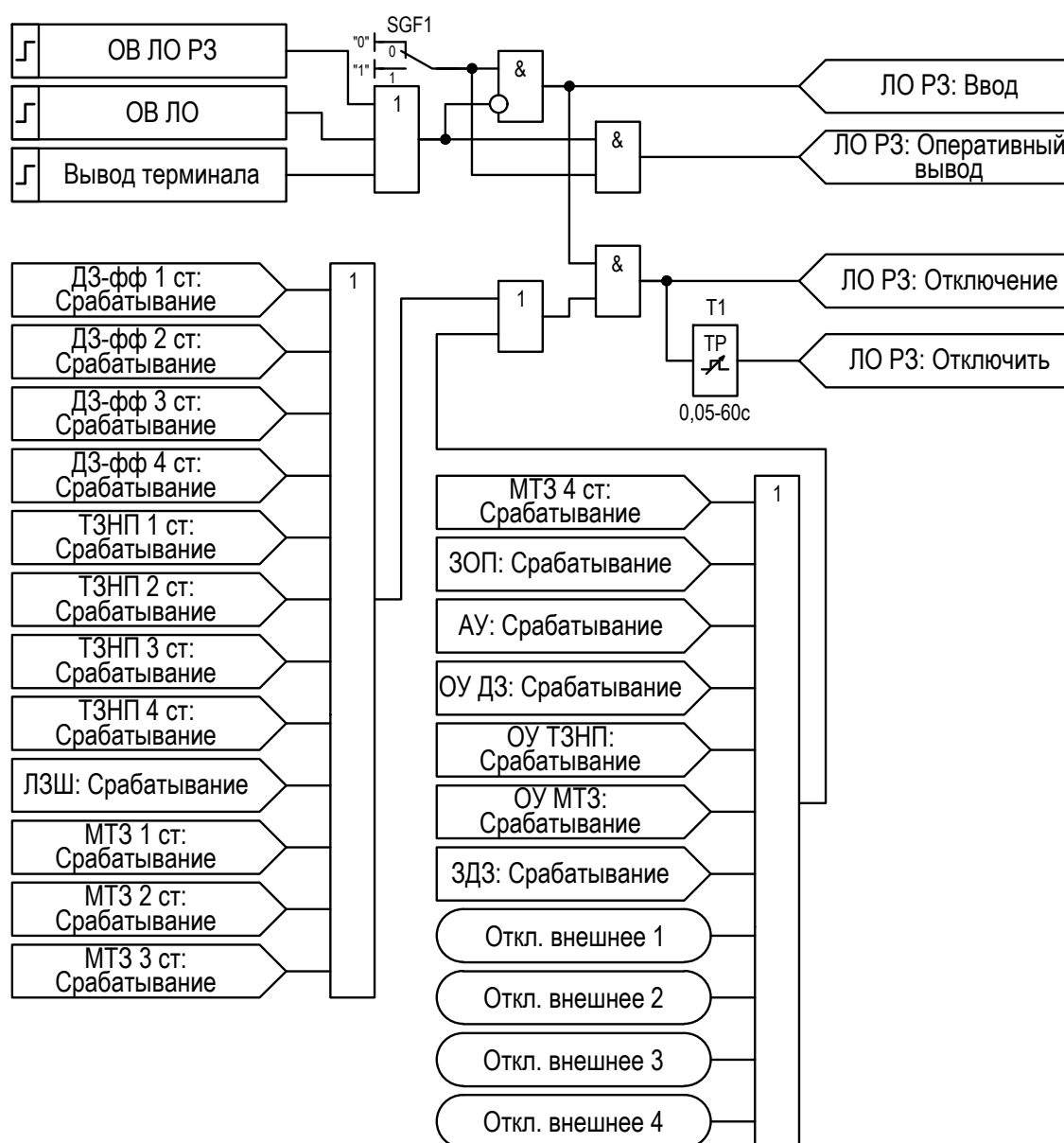
Рисунок 2.43 – Функциональная схема «ЛО РЗ»
