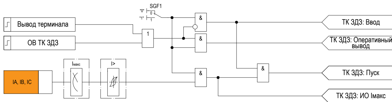
Рисунок 2.26 – Функциональная схема «ТК ЗД3»
