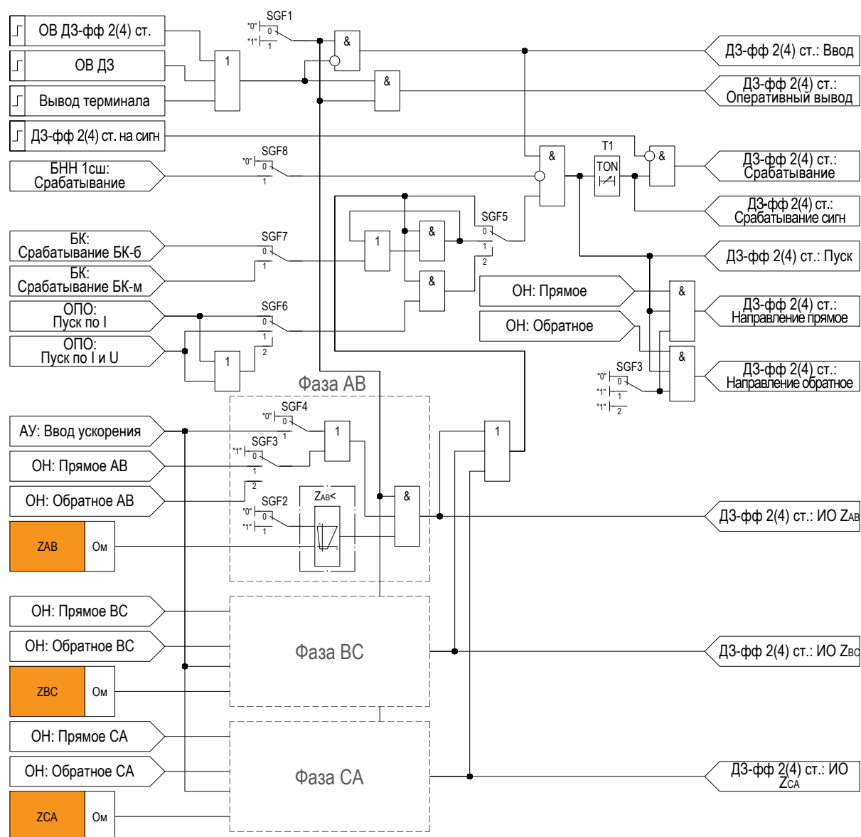
Рисунок 2.4 – Функциональная схема «ДЗ-фф 2(4)ст.»
