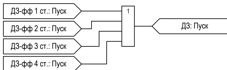
Рисунок 2.11 – Функциональная схема внешней логики ДЗ
