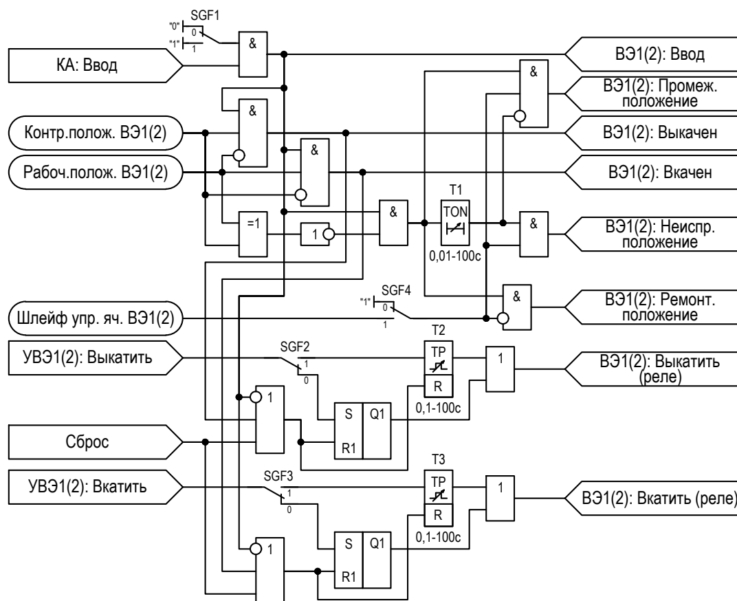
Рисунок 2.60 – Функциональная схема «ВЭ1(2)»
