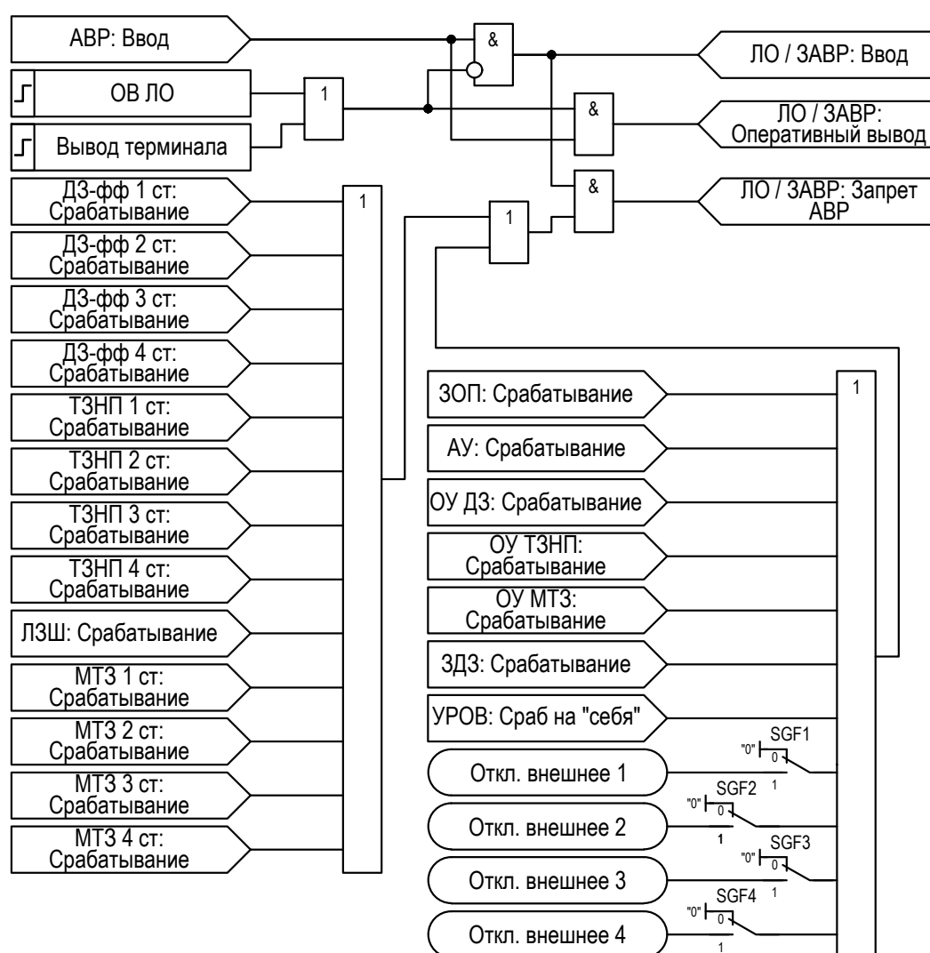
Рисунок 2.45 – Функциональная схема «ЗАВР ЛО»
