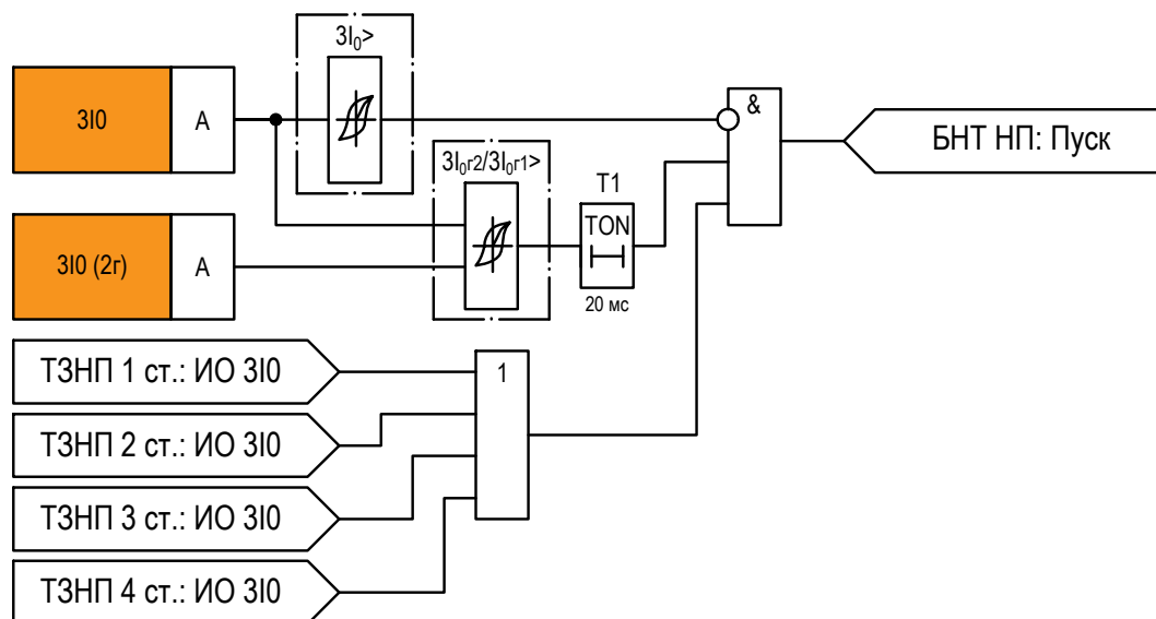
Рисунок 2.31 – Функциональная схема «БНТ НП»
