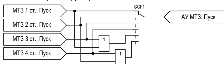
Рисунок 2.21 – Функциональная схема АУ МТЗ
