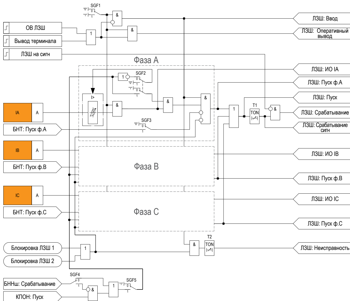
Рисунок 2.24 – Функциональная схема «ЛЗШ»
