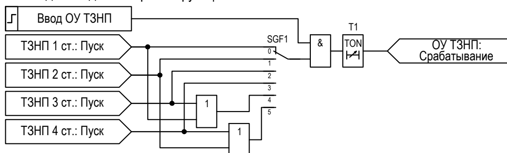
Рисунок 2.33 – Функциональная схема ОУ ТЗНП
