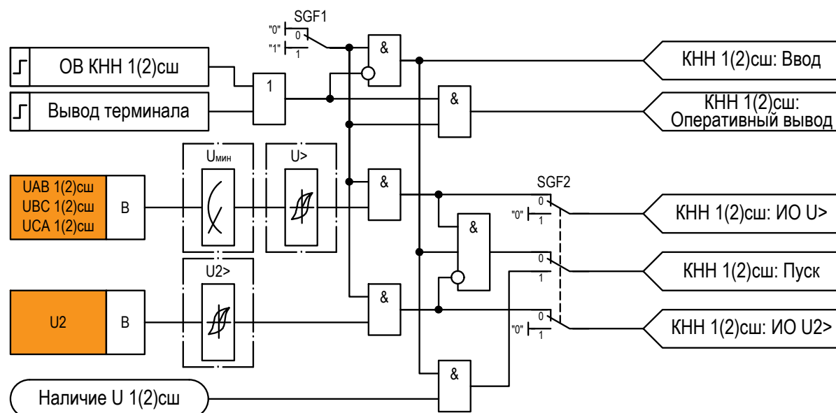
Рисунок 2.37 – Функциональная схема «КНН 1(2)сш»
