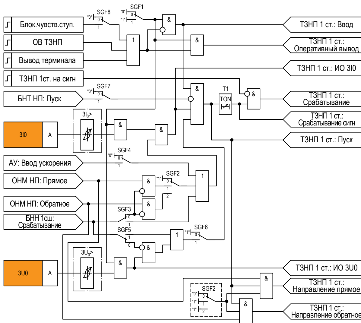
Рисунок 2.28 – Функциональная схема ступеней ТЗНП
