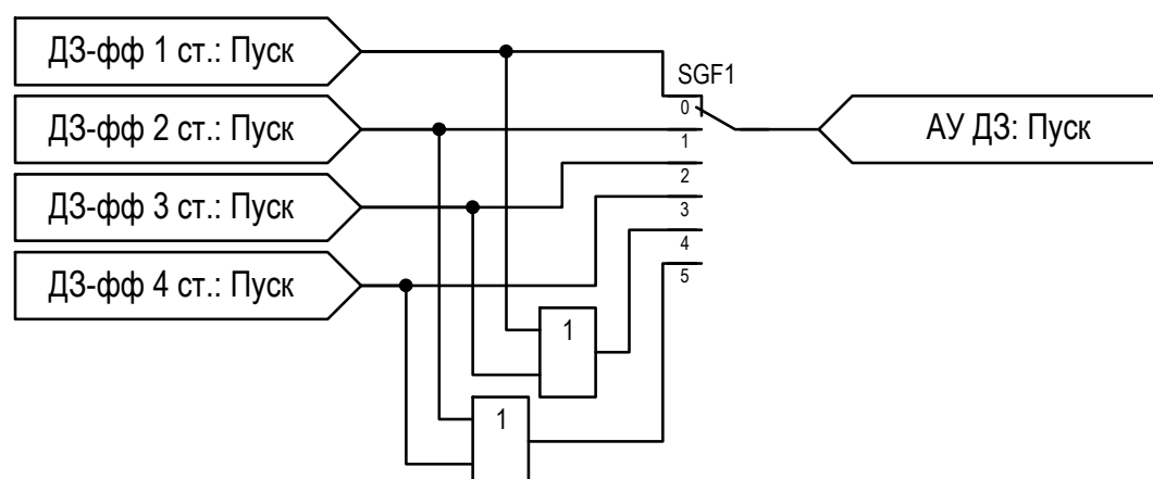
Рисунок 2.9 – Функциональная схема «АУ ДЗ»
