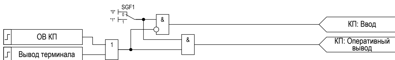
Рисунок 2.46 – Функциональная схема управления режимами работы функционального блока «КП»
