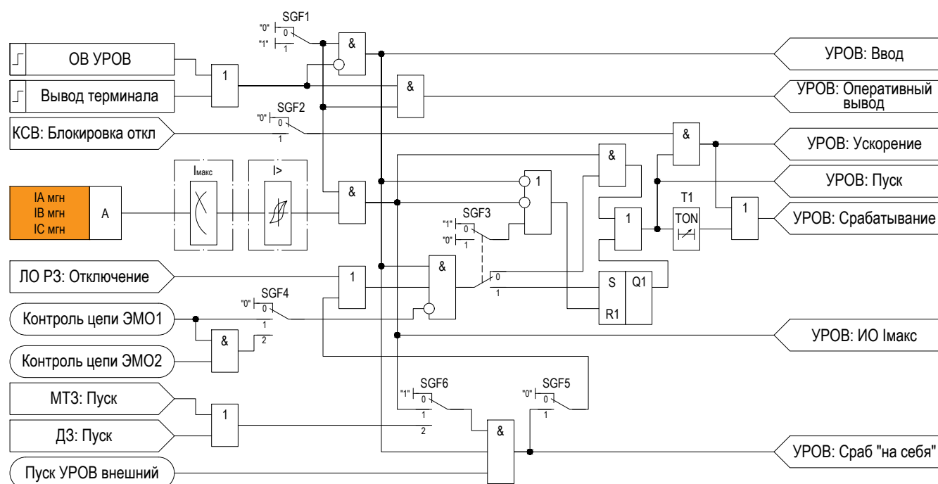
Рисунок 2.34 – Функциональная схема «УРОВ»
