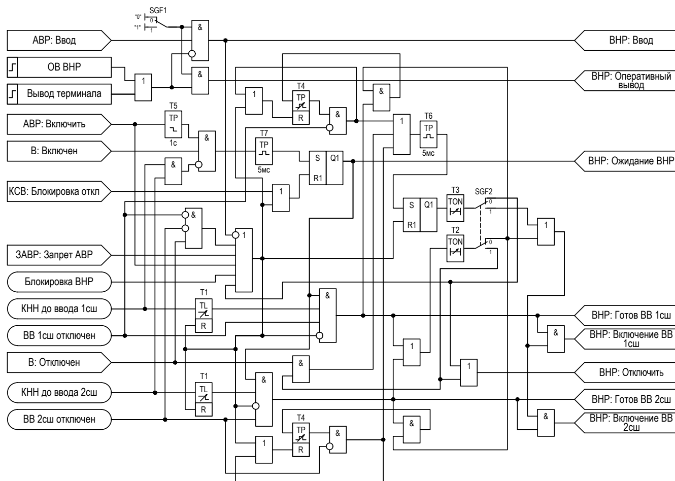
Рисунок 2.42 – Функциональная схема «ВНР»
