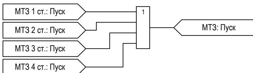
Рисунок 2.23 – Функциональная схема внешней логики МТЗ
