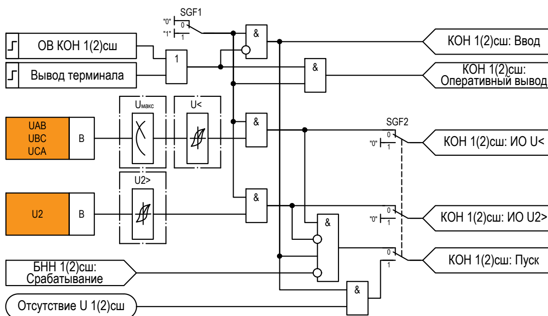
Рисунок 2.38 – Функциональная схема «КОН 1(2)сш»
