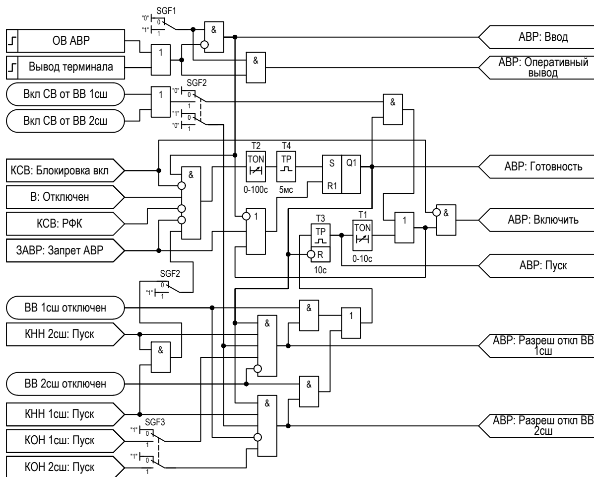
Рисунок 2.40 – Функциональная схема «АВР»
