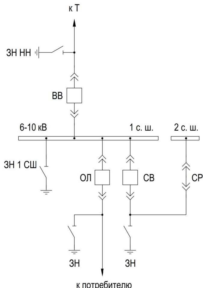
Рисунок 2.51 – Поясняющая схема первичной сети для алгоритмов оперативной блокировки КА
