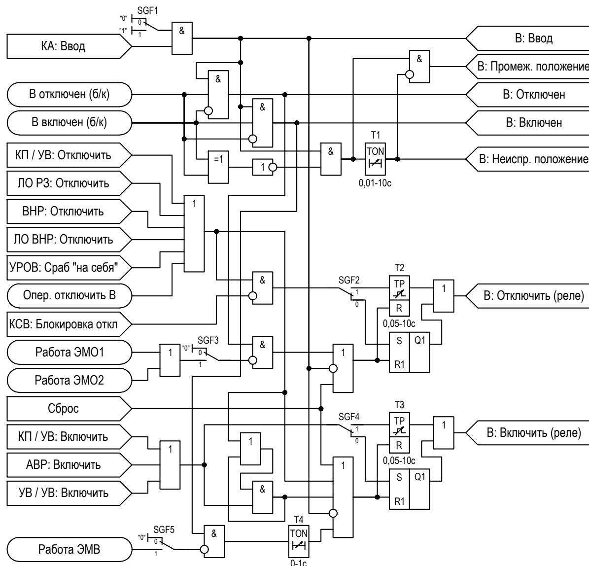
Рисунок 2.58 – Функциональная схема «Выключатель»
