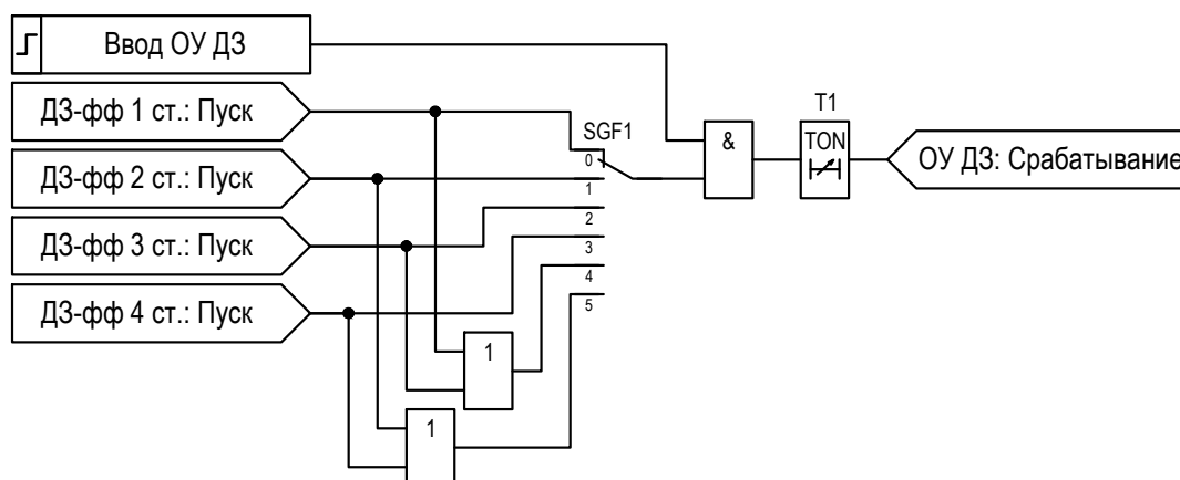
Рисунок 2.10 – Функциональная схема «ОУ ДЗ»
