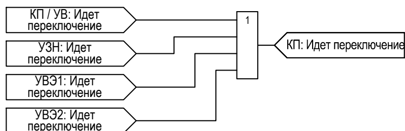
Рисунок 2.47 – Функциональная схема формирования общего сигнала переключения коммутационного аппарата
