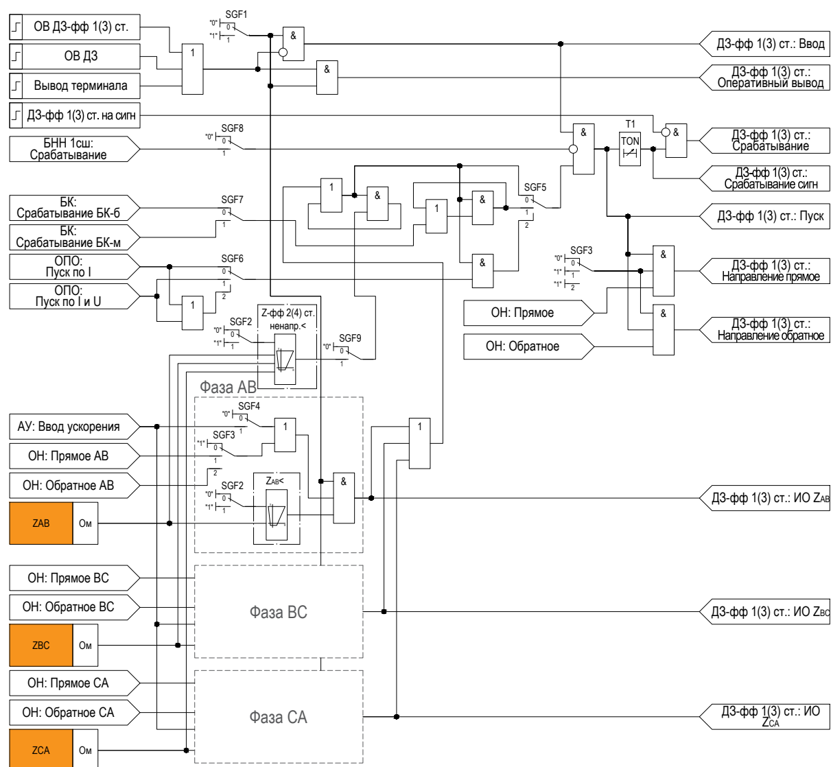
Рисунок 2.3 – Функциональная схема «ДЗ-фф 1(3)ст.»
