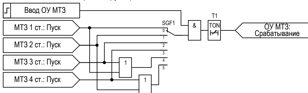
Рисунок 2.22 – Функциональная схема ОУ МТЗ
