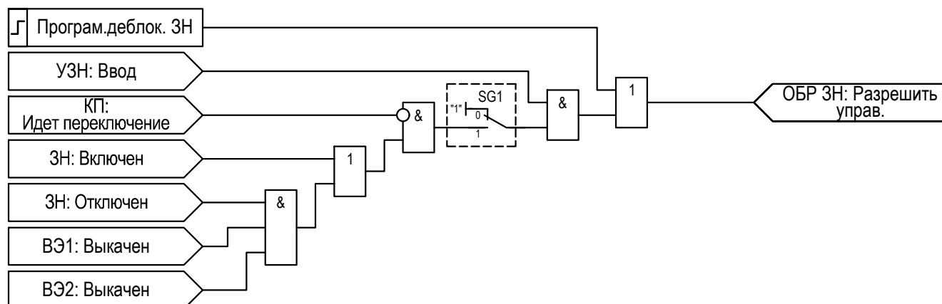
Рисунок 2.53 – Функциональная схема «ОБР ЗН»
