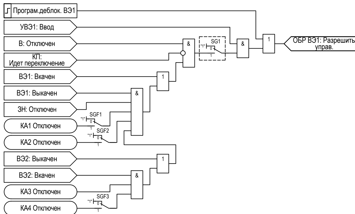
Рисунок 2.54 – Функциональная схема «ОБР ВЭ1»
