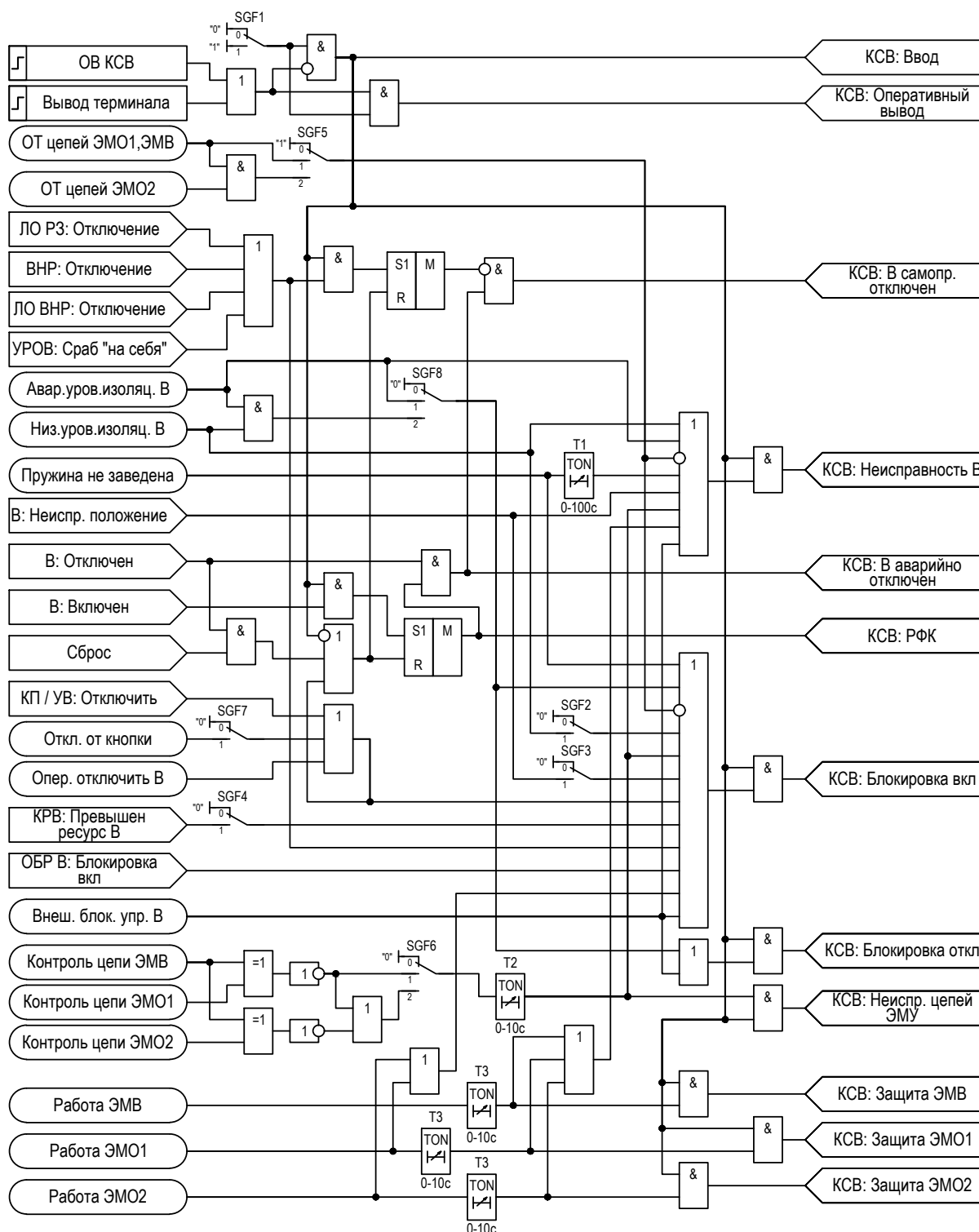
Рисунок 2.61 – Функциональная схема «КСВ»
