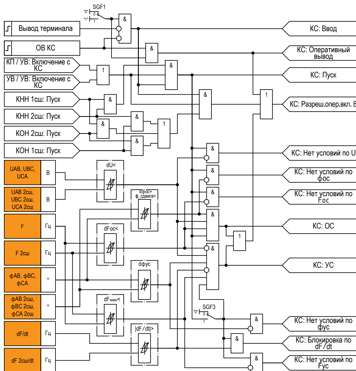
Рисунок 2.39 – Функциональная схема «КС»
